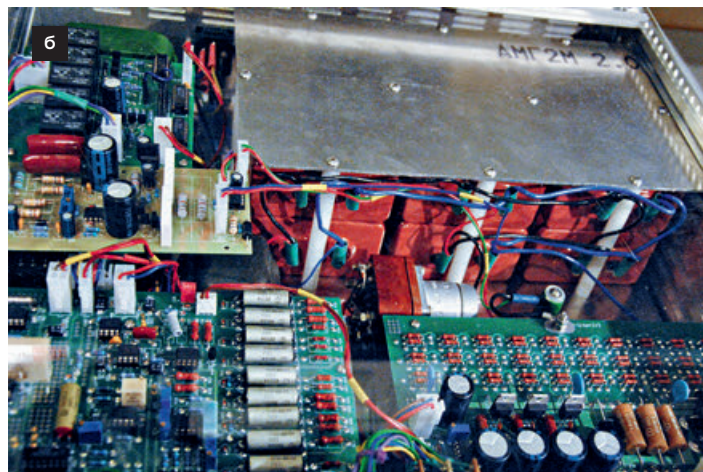
Генератор импульсов тока Г6-51/2 – одна из восьми моделей линейки Г6-51/Х, предназначенной для испытания защитных приборов мощными импульсами тока: а – общий вид выставочного образца; б – под панелью у задней стенки корпуса можно видеть группу конденсаторов с максимальным током разряда 4 000 А
